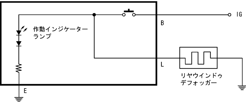
回路図
