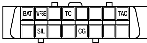
端子配列
