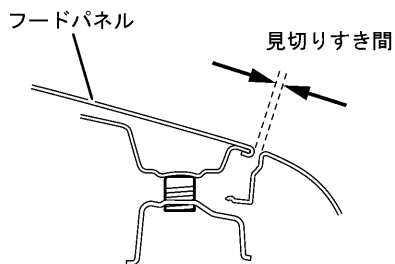
B-B 断面
