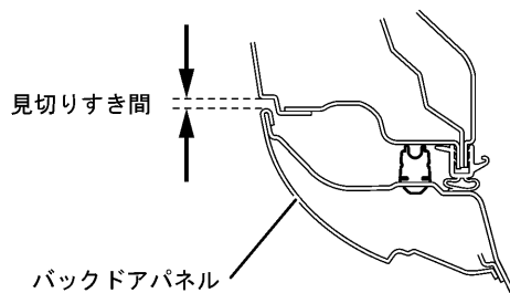
C-C 断面
