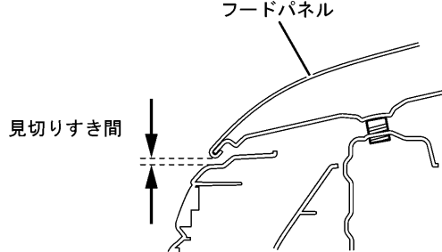
A-A 断面
