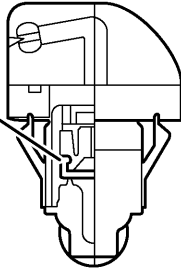
リヤウォッシャーノズル断面
