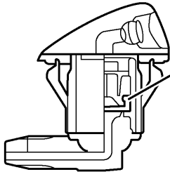
フロントウォッシャーノズル断面
