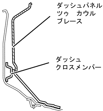
A-A 断面
