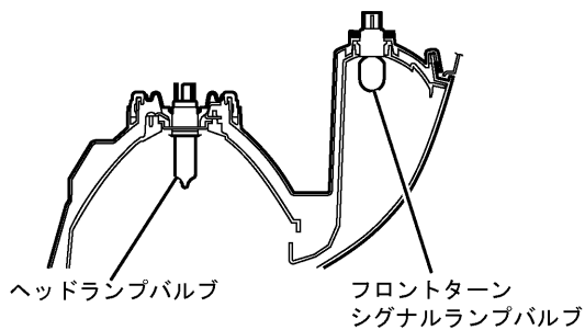
C-C断面
