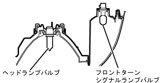
A-A断面
