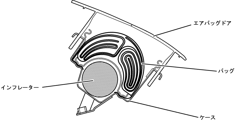
助手席SRSエアバッグASSY断面
