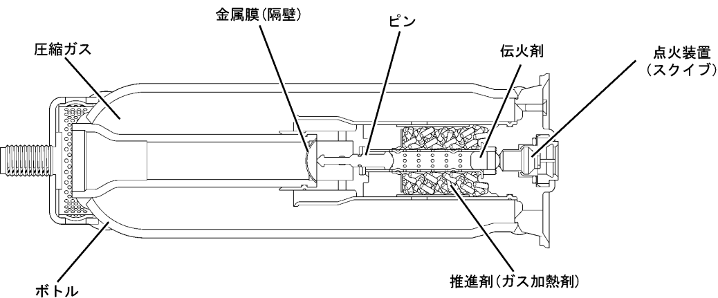
インフレーター断面
