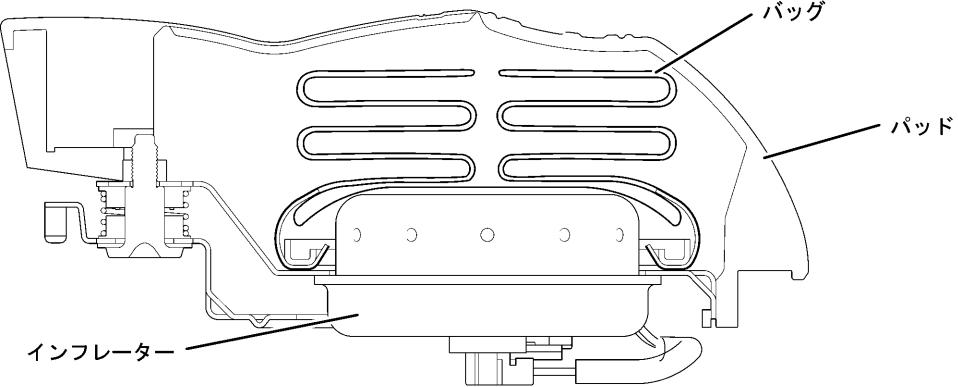
運転席エアバッグASSY
