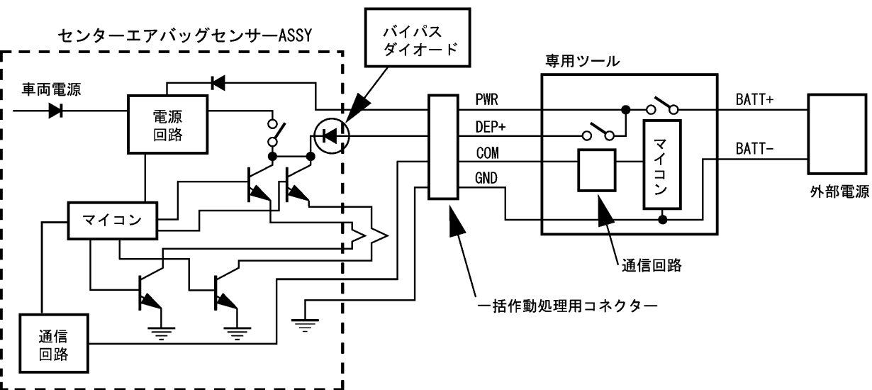
一括作動処理回路
