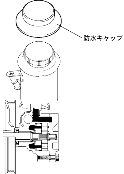
ペーンポンプ & リザーバー
