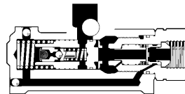
フローコントロールバルブ断面
