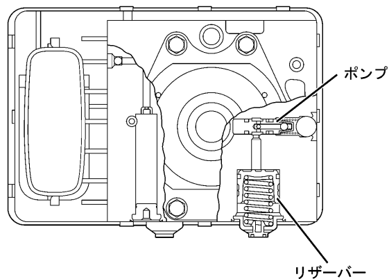
C視断面
