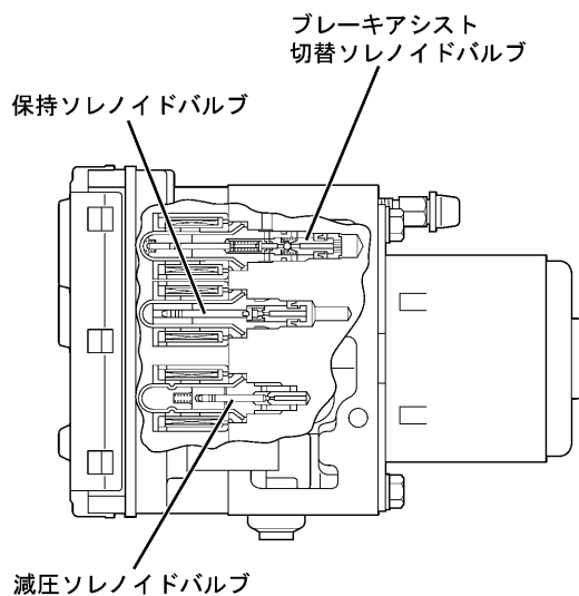
B視断面
