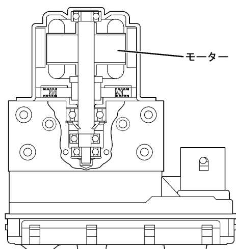
A視断面
