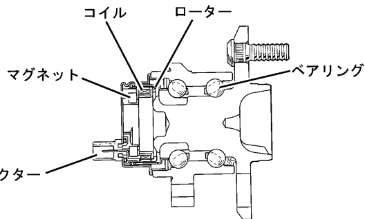
アクスルハブベアリングユニット
