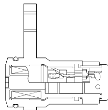
車輪速センサー断面
