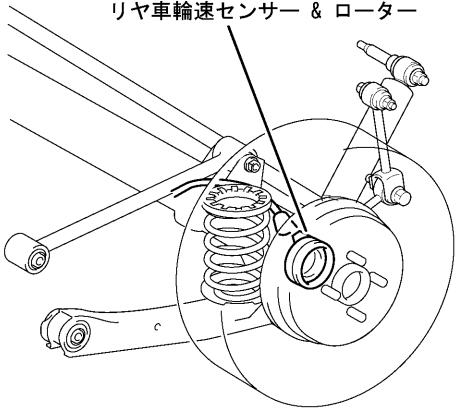
センサー配置
