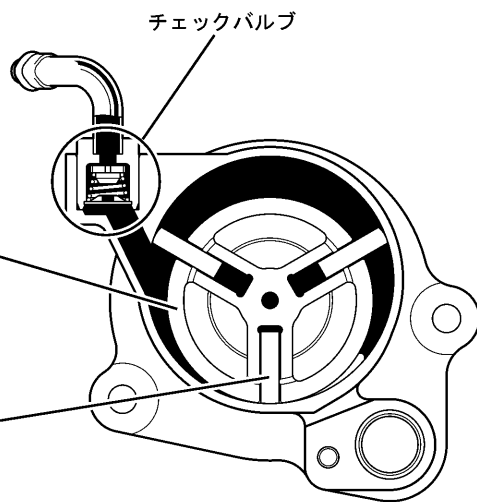
B-B' 断面
