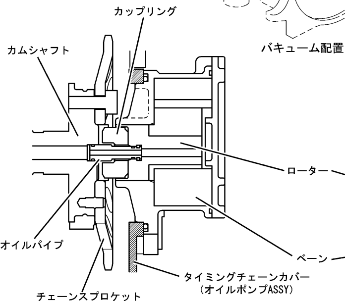
A-A' 断面
