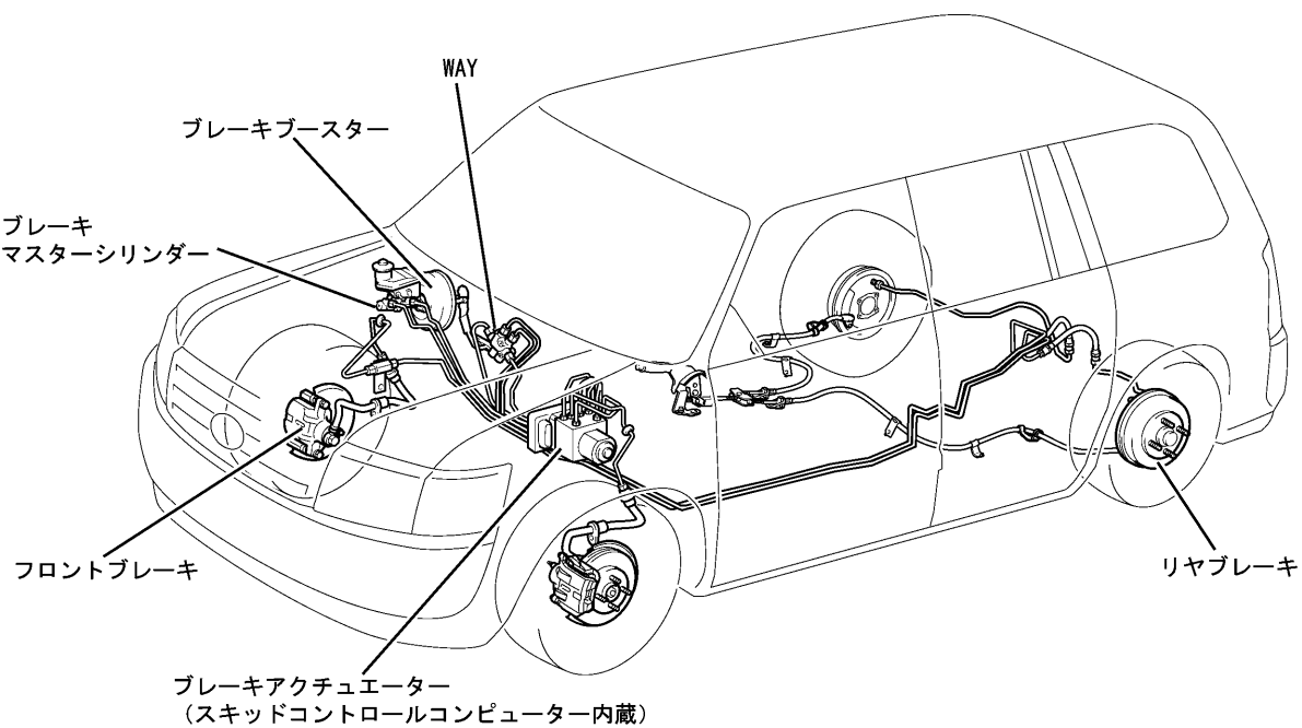
4WD (ABS付き) 車
