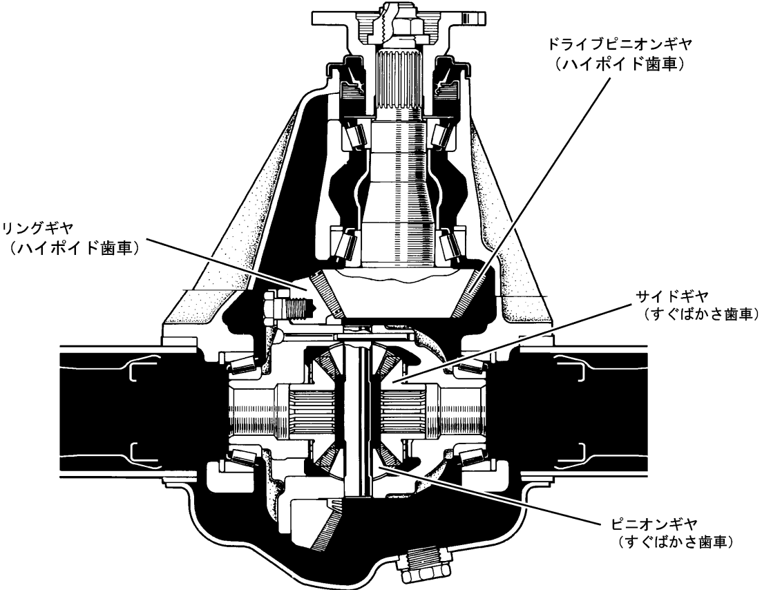
リヤディファレンシャル
