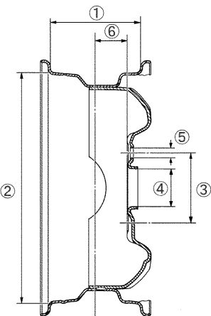
13×5Jスチールホイール (シルバー色・ブラック色)
