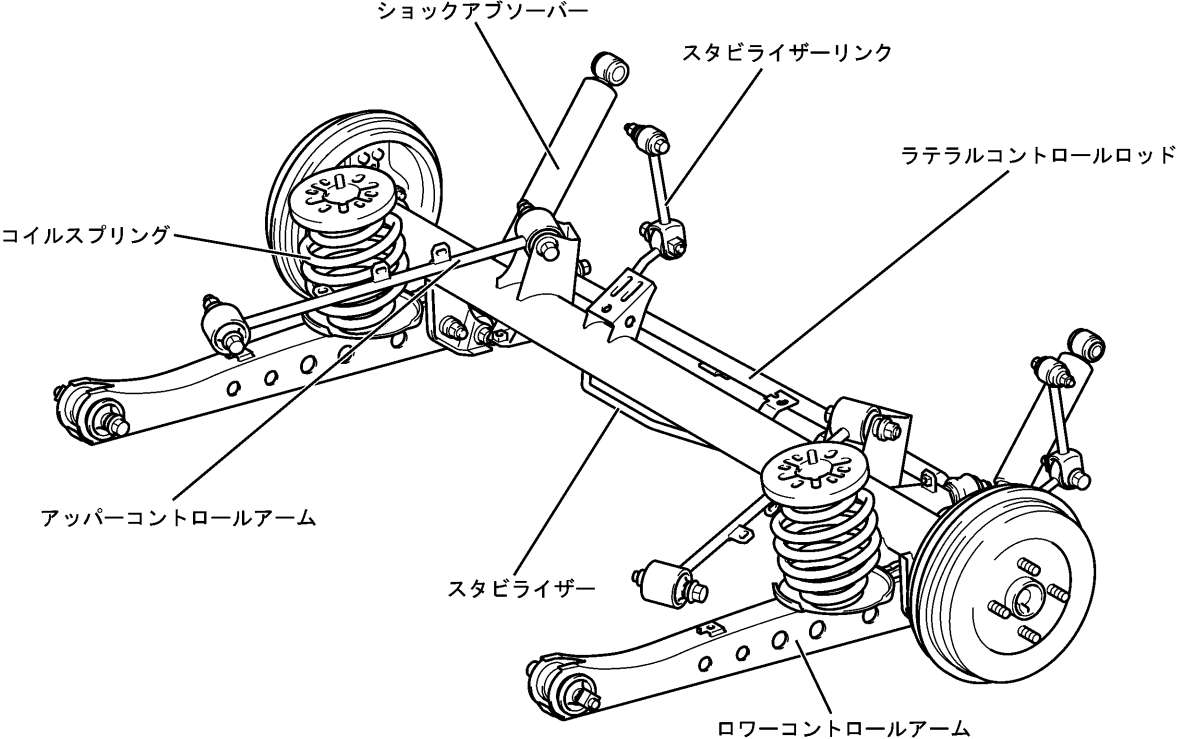
リヤサスペンション (2WD車)
