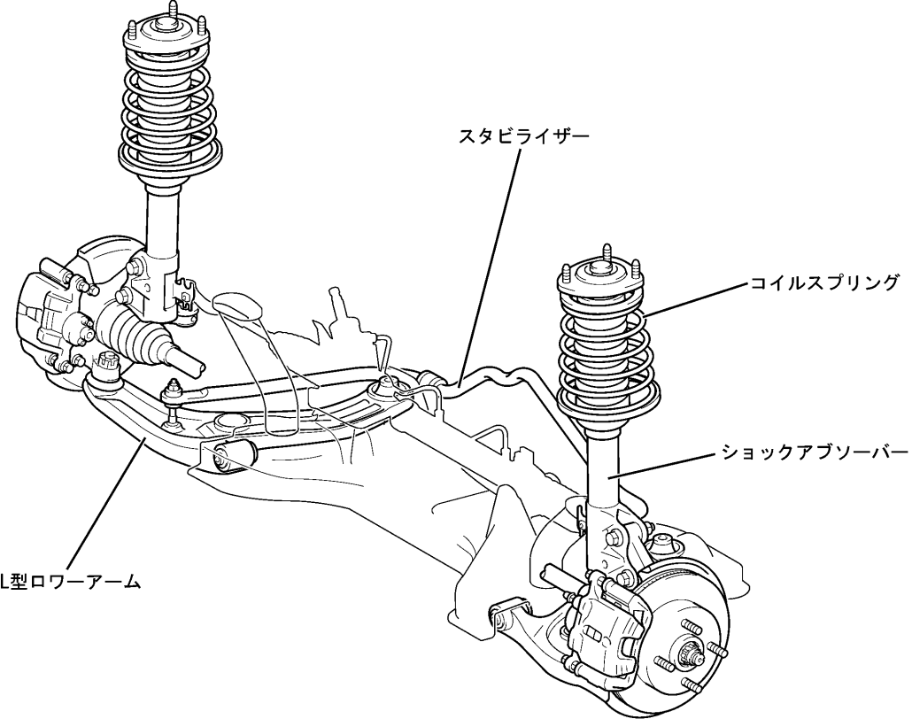
フロントサスペンション (4WD車)
