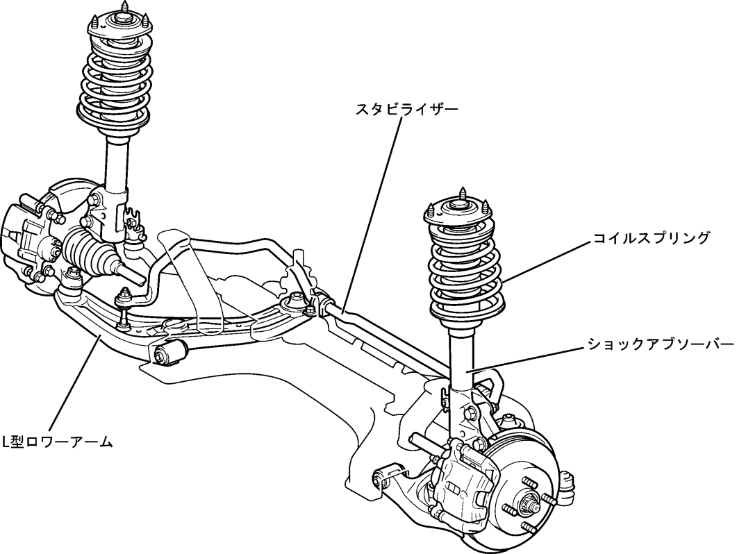
フロントサスペンション (2WD車)
