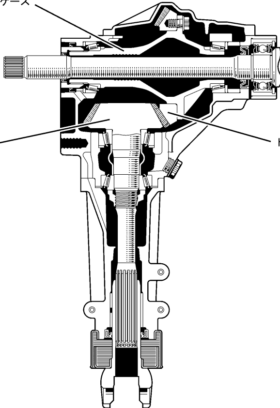
MF1A型トランスファー
