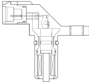
入力軸回転数センサー
