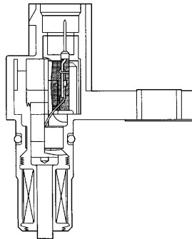
入力軸回転数センサー
