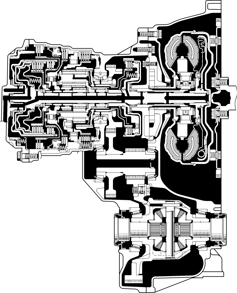
U441E型
