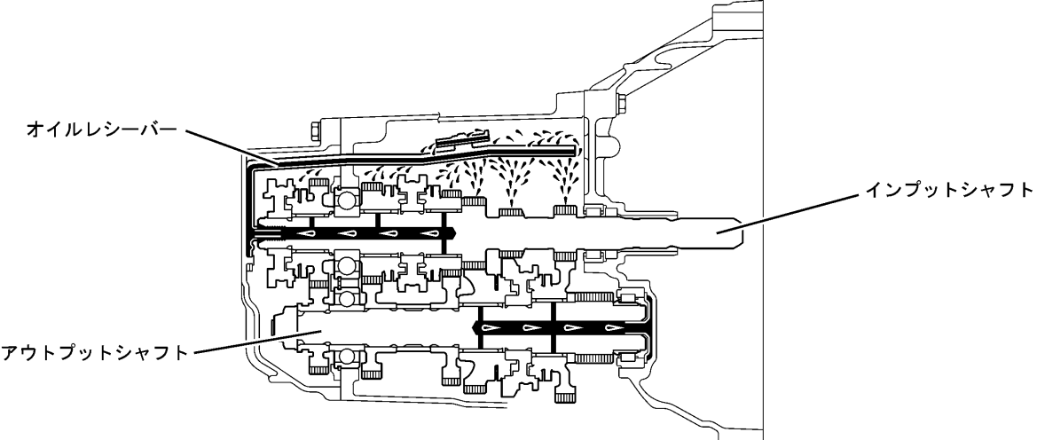
インプットシャフト関係の潤滑
