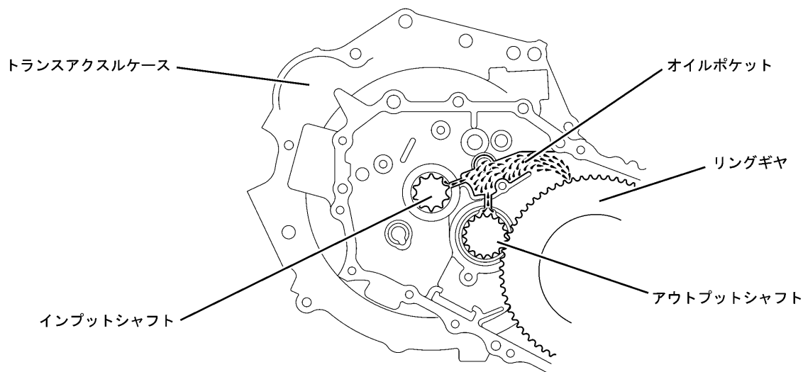
アウトプットシャフト関係の潤滑
