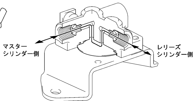
アキュムレーター立体断面
