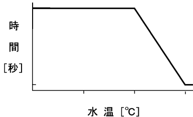
グローインジケータランプ 点灯時間特性
