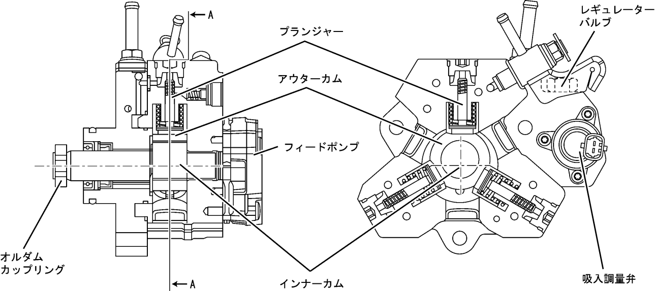
A-A断面
