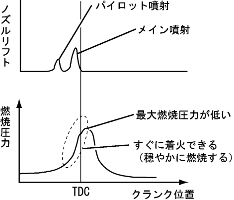
パイロット噴射有り
