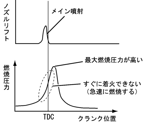
〈参考〉パイロット噴射無し
