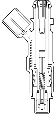
インジェクター断面
