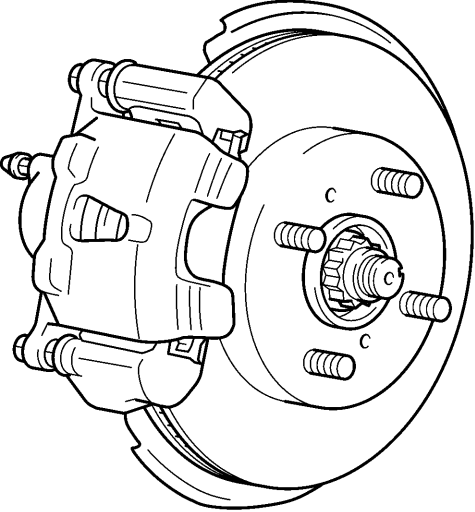
フロントブレーキ（13" タイプ）
