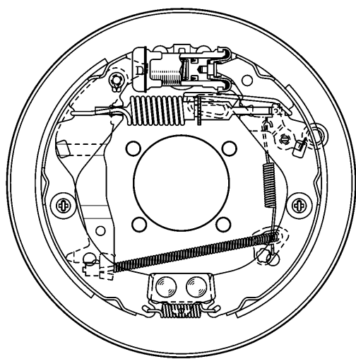
リヤブレーキ（228LT型）
