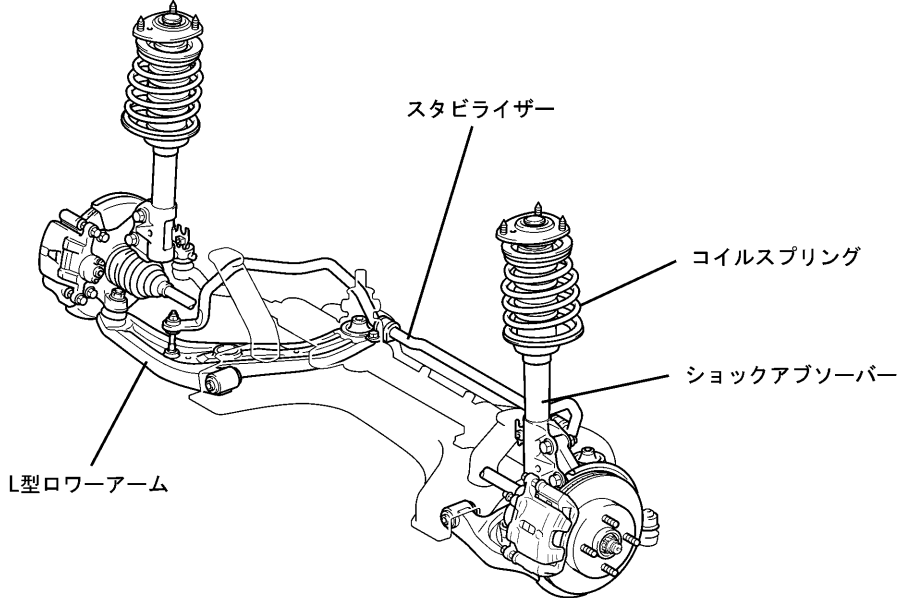
フロントサスペンション
