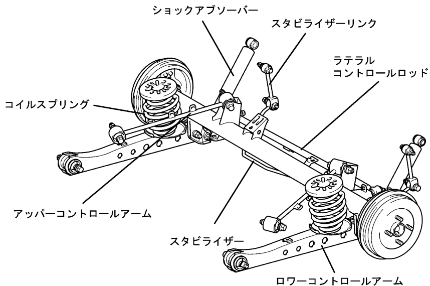
リヤサスペンション
