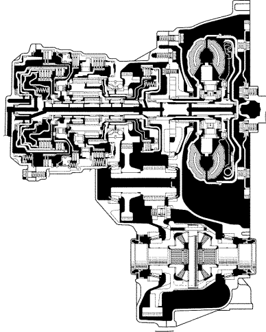
U441E型オートマチック トランスアクスル
