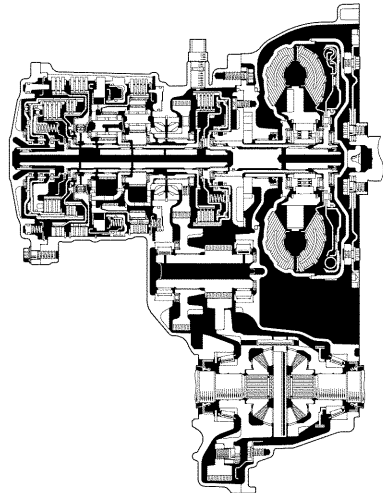
U340E型オートマチック トランスアクスル RAA0412S
