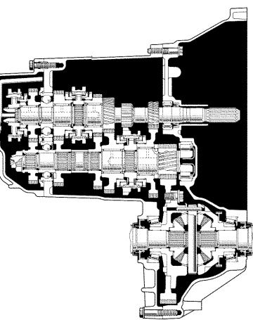
C5#型マニュアル トランスアクスル
