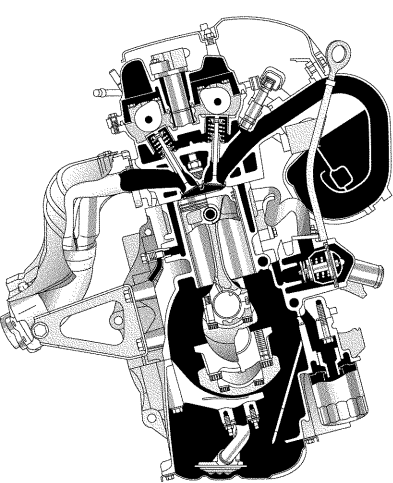
2NZ-FEエンジン
