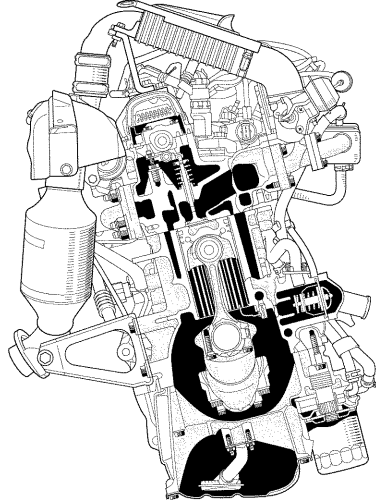
1ND-TVエンジン
